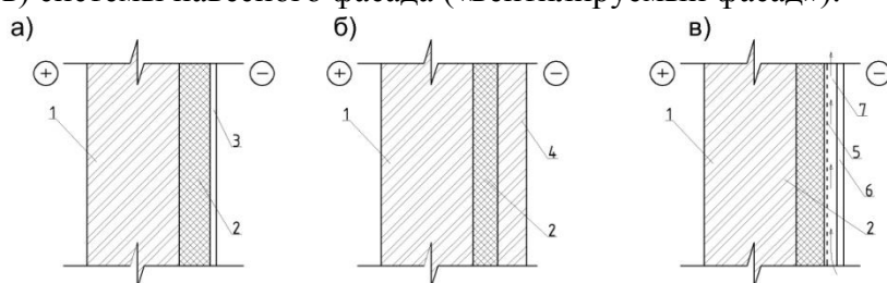
Рис. 1 – Основные конструктивные типы наружных стен
