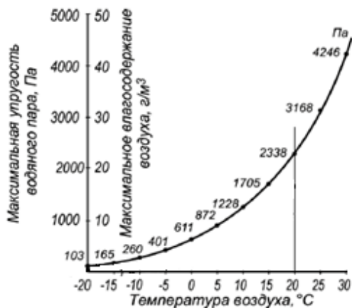
Рис.3. Зависимость максимальной упругости водяного пара E (Па) от температуры воздуха ( ^\circ\text{C} )
