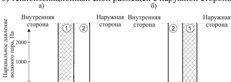
Рис.2. Два варианта расположения слоев в ограждающей конструкции
